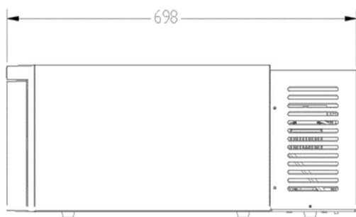
Wymiary zewnętrzne oraz zbiornika lodówki WERTBERG LS 5.32
